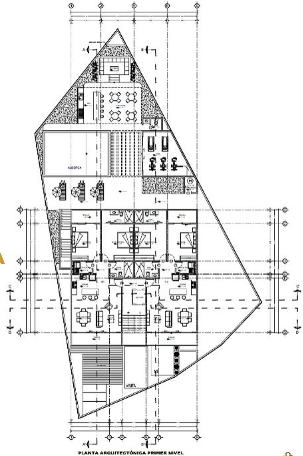
PLANTA ARQUITECTÓNICA PRIMER NIVEL
